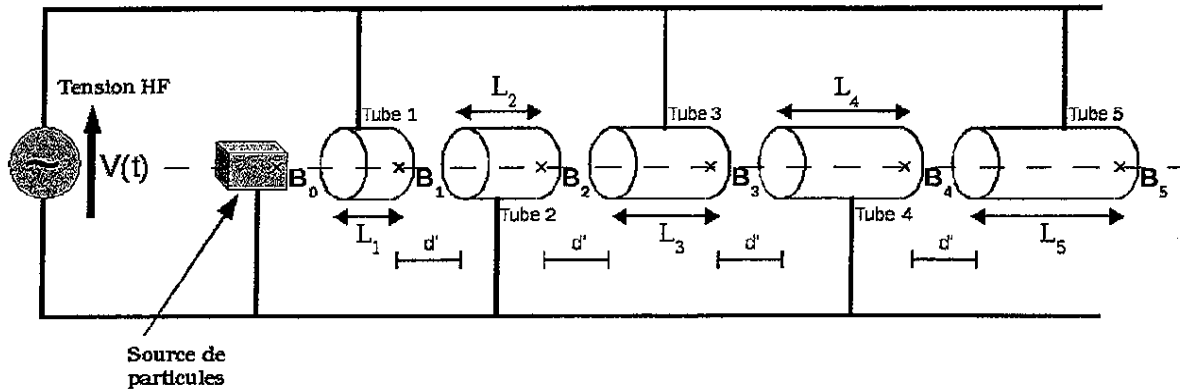
FIG. III.3 – Accélérateur de WILDERÖE
