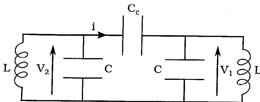
FIG. III.6 – Modèle électrique pour deux cavités idéales couplées
