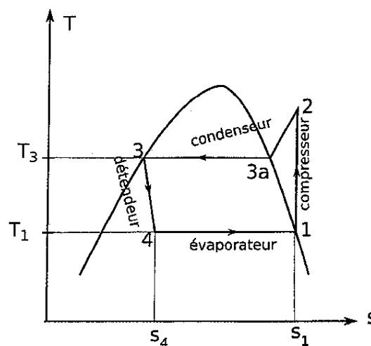
FIG. II.4 – Allure du diagramme entropique du R\ 717 , l'entropie massique est placée en abscisse et la température en ordonnée. On a représenté la courbe d'équilibre liquide-vapeur et les étapes du cycle.
